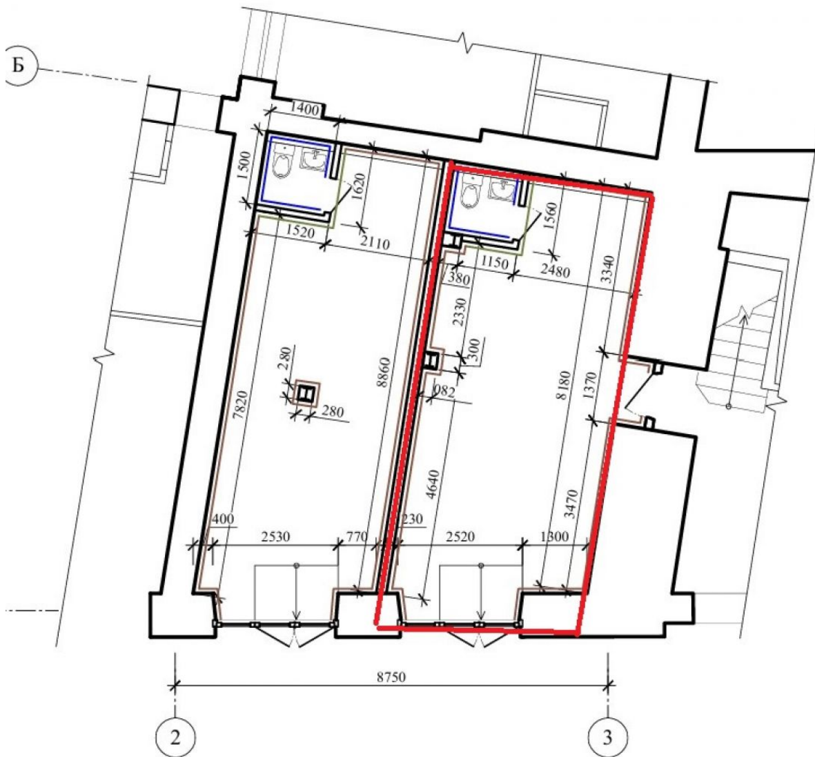
План перегородок помещения 1 по плану № 04/001/2017
